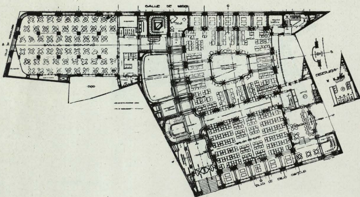
PLANTA BAJA.
