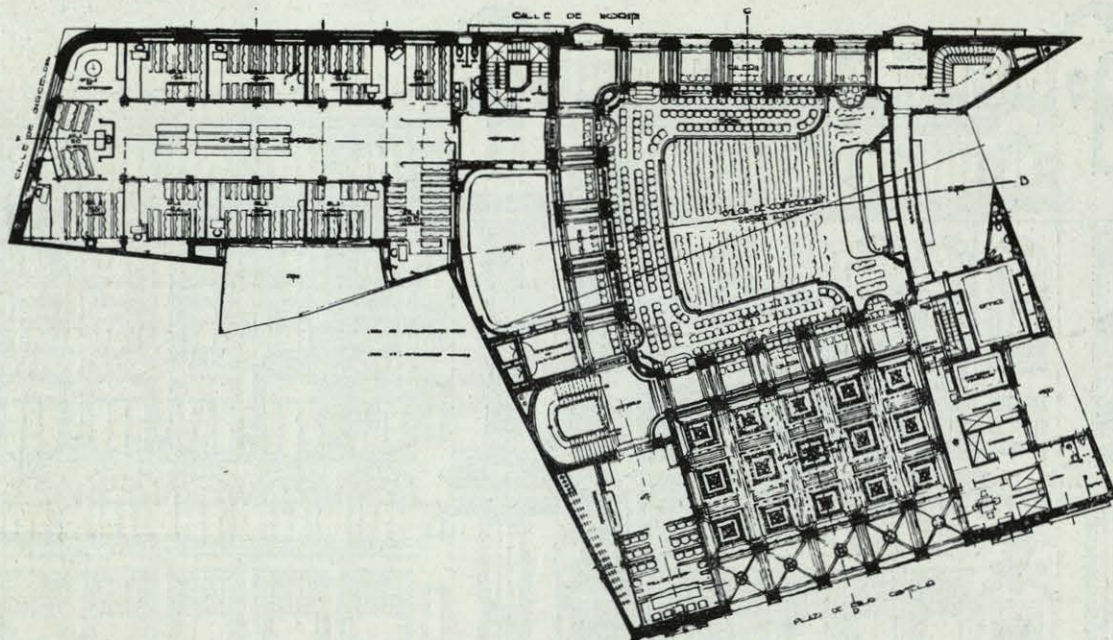
PLANTA PRINCIPAL.
